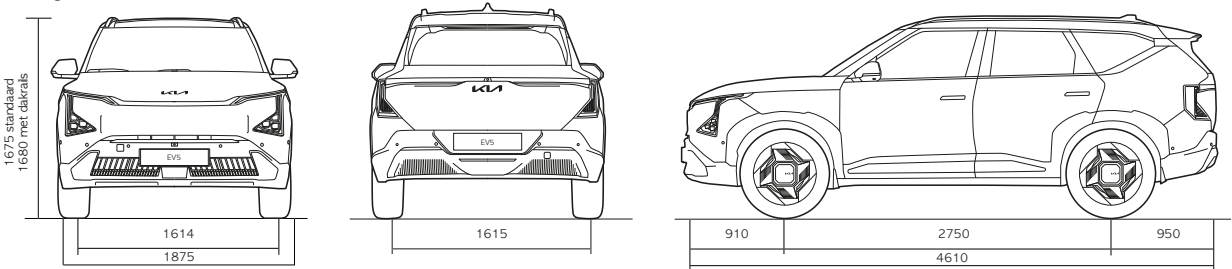
Afmetingen GT-Line
